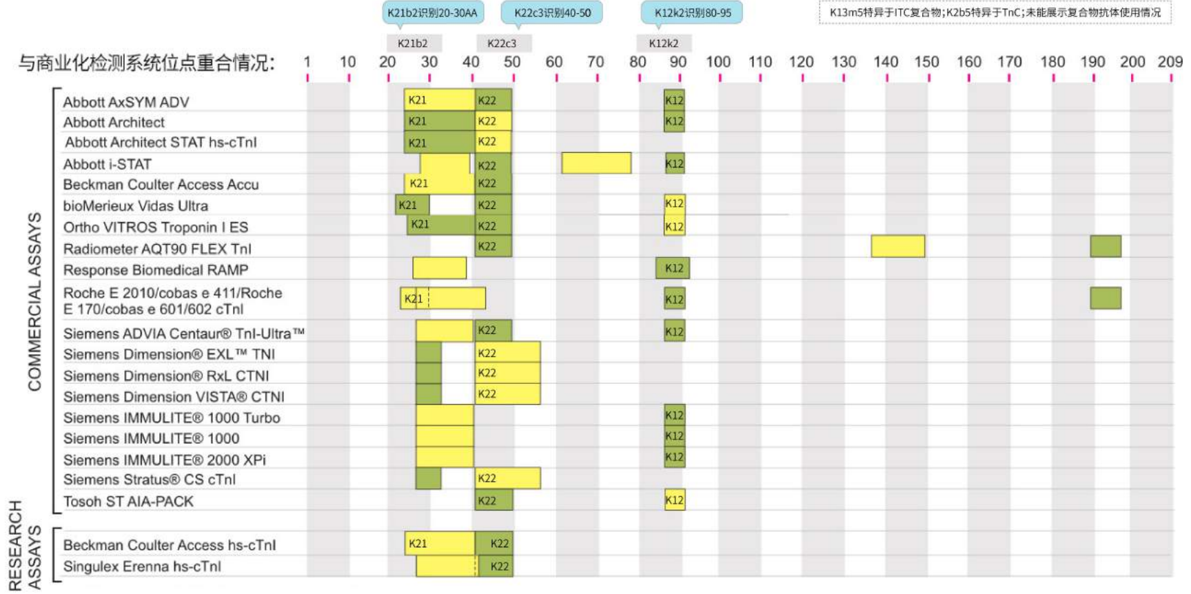
图 8. 商品化的 cTnI 免疫检测系统中使用的抗体表位。绿条和黄条分别代表捕获抗体和检测抗体的识别位点。此图基于国际临床化学联合会 (IFCC) 网站 www.ifcc.org 中所提供的信息 (Scientific Division > SD Documents > Troponin assay analytical characteristics.)。
